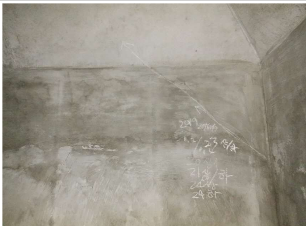
유입배관실 벽체 균열(0.3mm미만)
