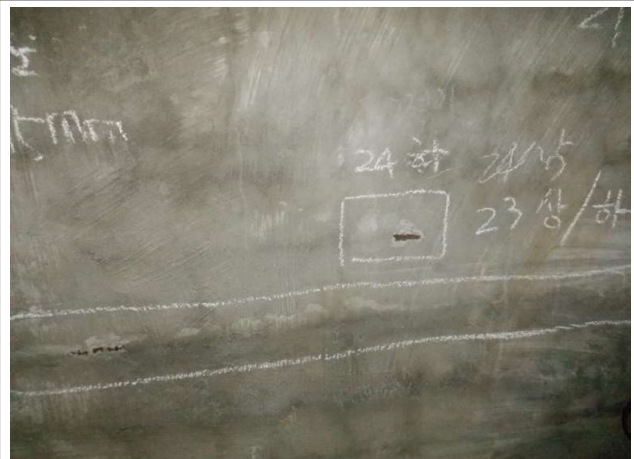
유입배관실 벽체 철근노출, 박락
